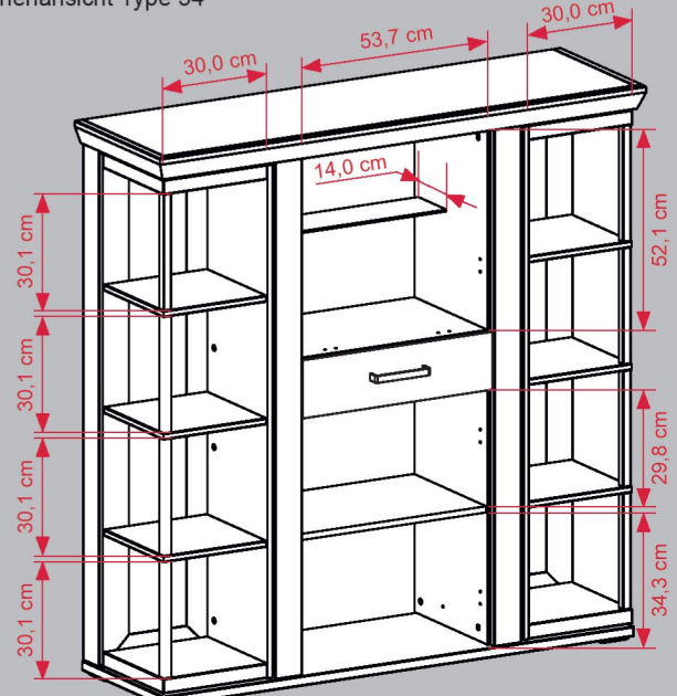
Innenansicht Type 54
