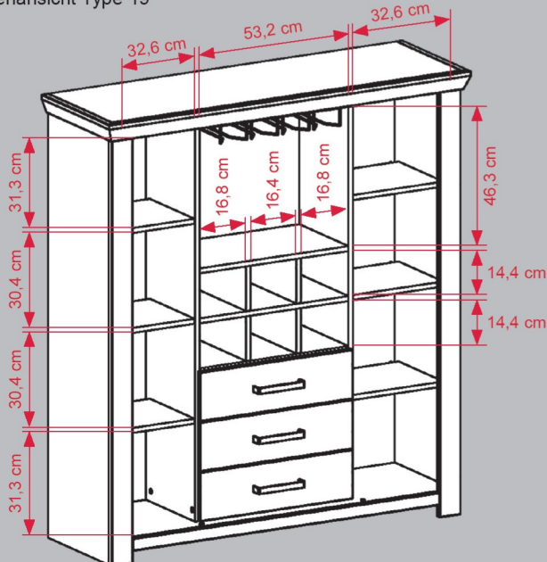
Innenansicht Type 19
